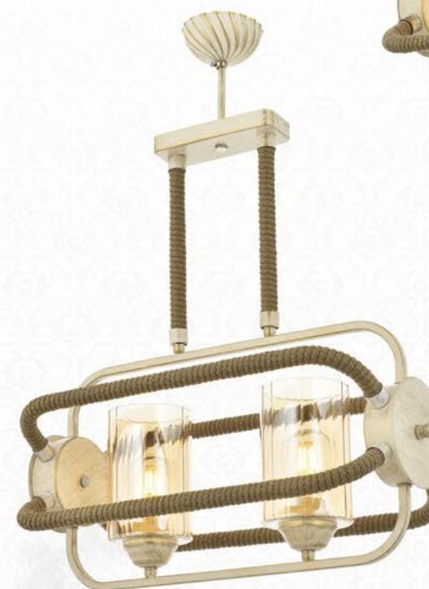
2001-2 W:50x25 H:65 2 x E27 Max.60W
